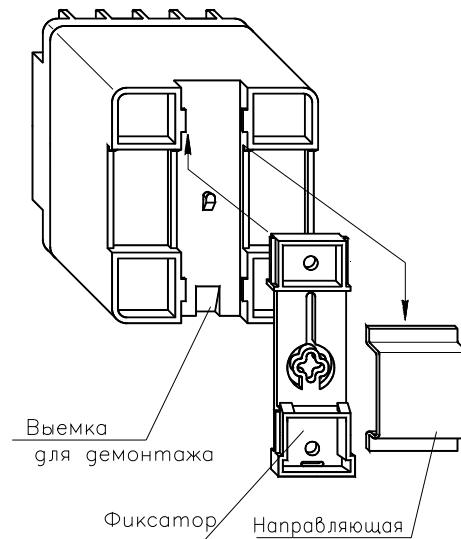
Рисунок В.1 Вариант крепления на направляющую
